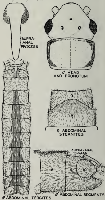
Fig. 86.— Alloperla occidentis .
