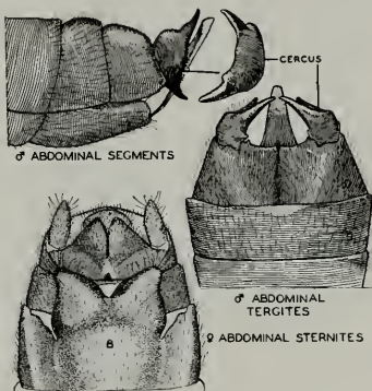
Fig. 72.— Leuctra forcipata .
