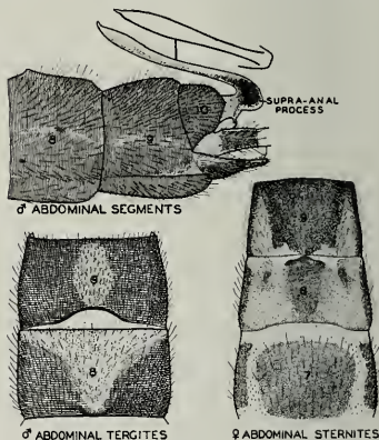
Fig. 77.— Capnia promota .
