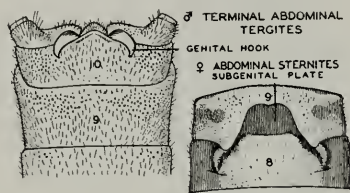
Fig. 64.— Acroneuria evoluta .
