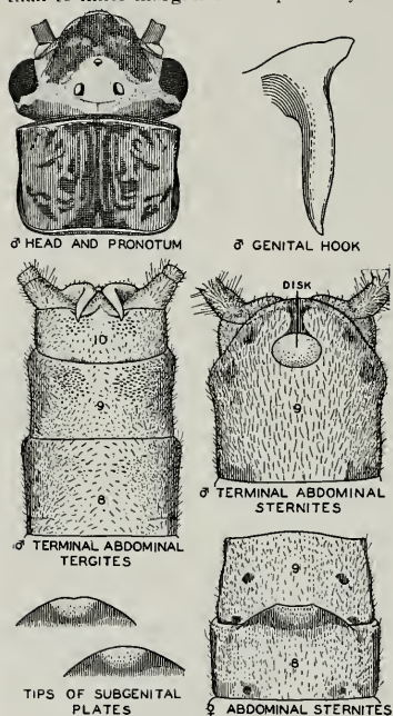
Fig. 65.— Acroneuria perplexa .
