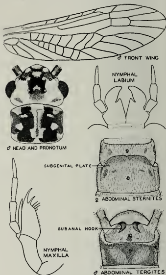
Fig. 81.— Isoperla pinta .
